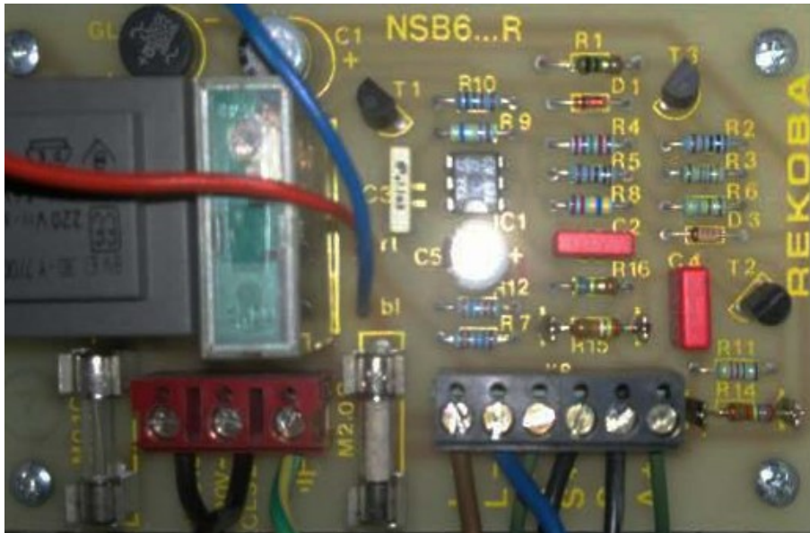
NSB6..R - Platine
